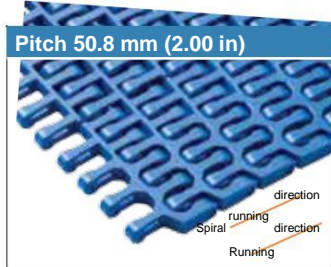
uni Flex L-ASB Strength Index (POM)
